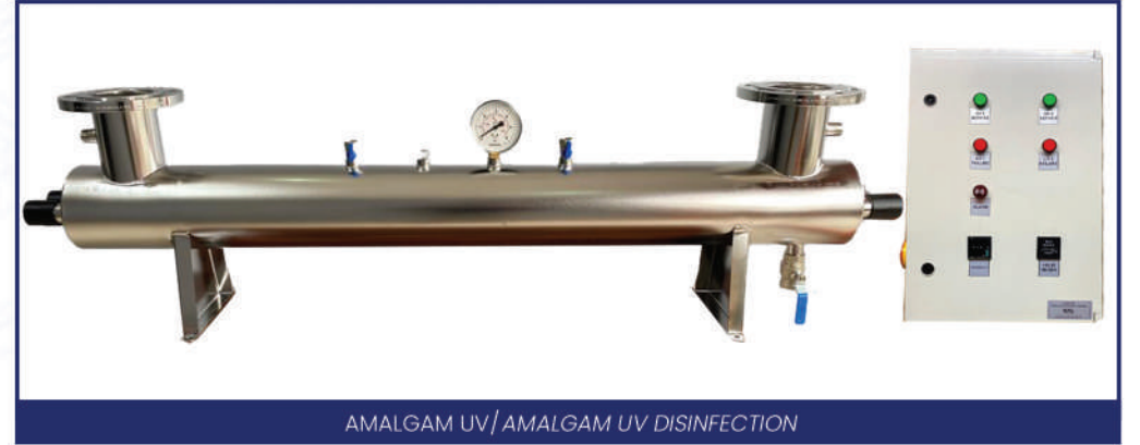
PASLANMAZ FİLTRE KABİ STAINLESS STEEL
